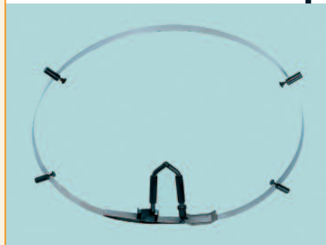
Innenumfangsband IUB mit Spreizzange und 4 Werkstückauflagen
