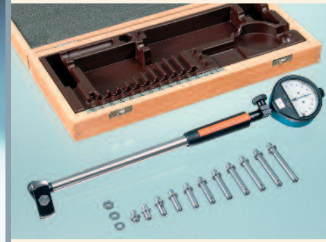
SUBITO® SU 50 - 100
